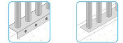
Base en U atornillada
